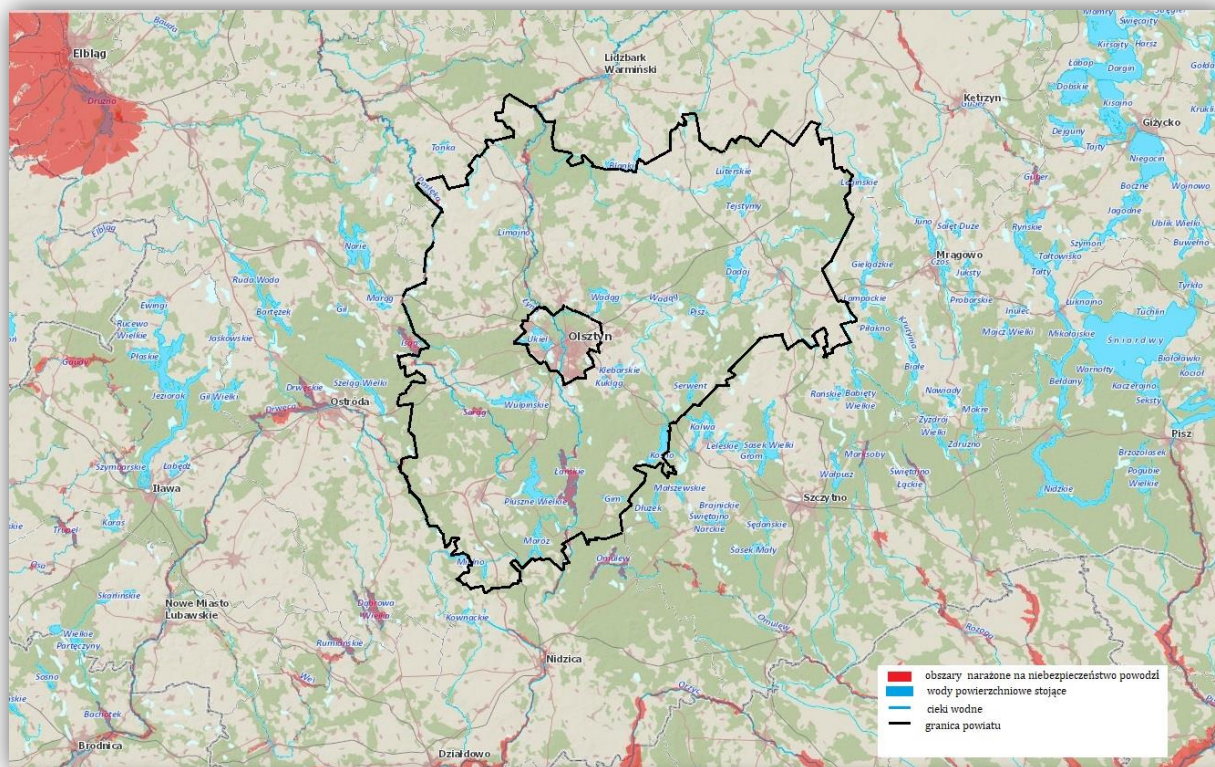
Mapa 9. Obszary narażone na niebezpieczeństwo powodzi na terenie powiatu olsztyńskiego Źródło: https://wody.isok.gov.pl/imap_kzgw/?gpmmap=gpWORP dostęp dnia 14.07.2021
